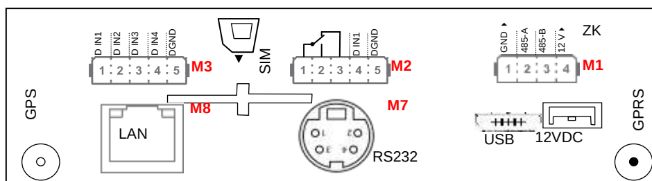
Steckerbelegung des EVO 2.8 Pure V4
